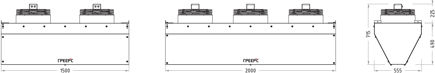
ГРЕЕРС ЗВП-М1-150/200Н:
