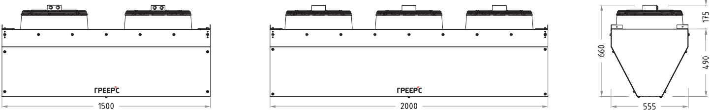
ГРЕЕРС ЗВП-М2-150/200Н:
